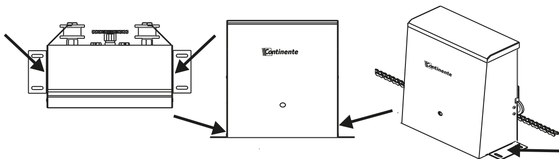
Figura 02: Fixar as base do Movimentador Deslizante
